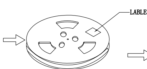
② 卷盘贴标签示意图
