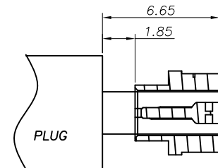
对插示意图
