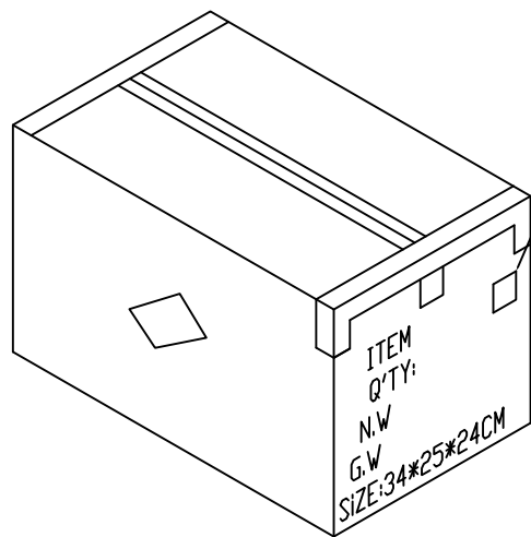
外箱封口“工”字型, 一箱数量512pcs, 16盘.
