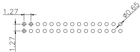
P.C.Board Layout
