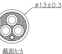
截面A-A
