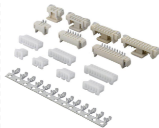
1.25mm 线对板 A1251系列
