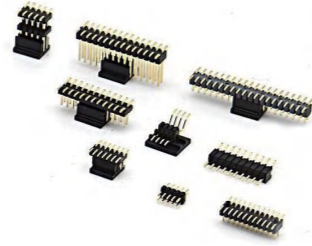
1.27mm 排针 PH1276系列
