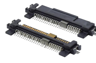
8639 3.0 PCI+SAS 8000系列
