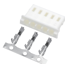
2.50mm 线对板 12503系列
