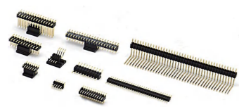
2.00mm 排针 PH2005系列
