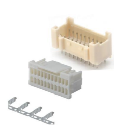
2.00mm 线对板 A2019系列
