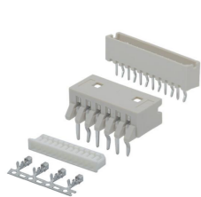
2.00mm 线对板 A2004系列
