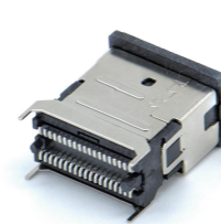
Slimsas 38P 4X 立式 贴板180°母座 80601系列
