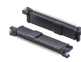
8639 3.0 PCI+SAS 80602系列
