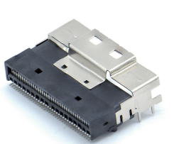
Slimsas 74P 8X 卧式 贴板90°母座 80601系列
