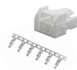
2.00mm 线对板12002系列带锁扣
