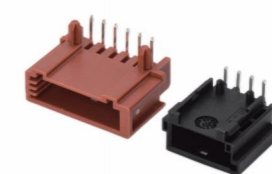
2.54mm 线对板 12540系列
