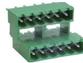
WLACXXX0S-XXF0007系列 5.0-5.08mm PIN数: 04-48P
