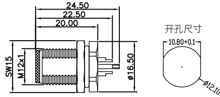
尺寸图 / Dimension
