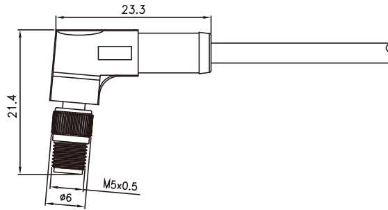
尺寸图 / Dimension
