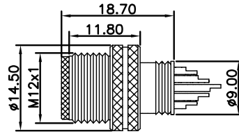
尺寸图 / Dimension
