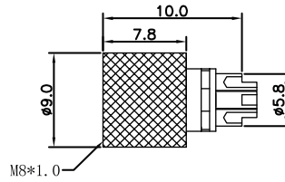
尺寸图 / Dimension
