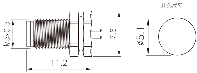
尺寸图 / Dimension
