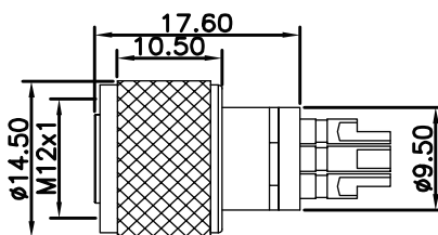
尺寸图 / Dimension
