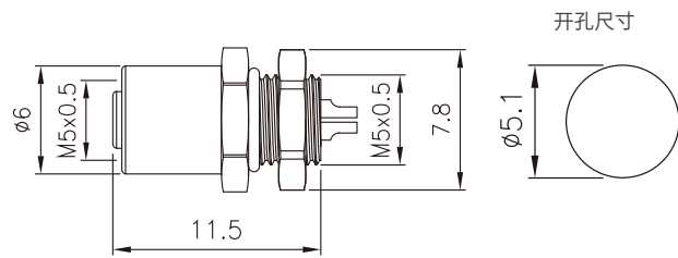
尺寸图 / Dimension
