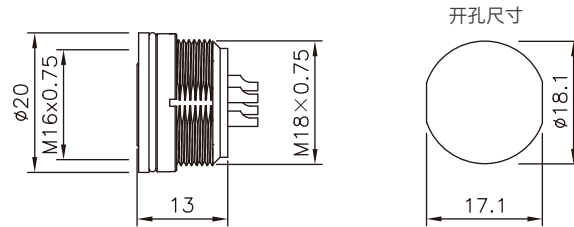
尺寸图 / Dimension
