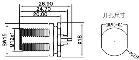
尺寸图 / Dimension
