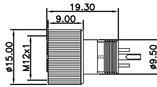
尺寸图 / Dimension
