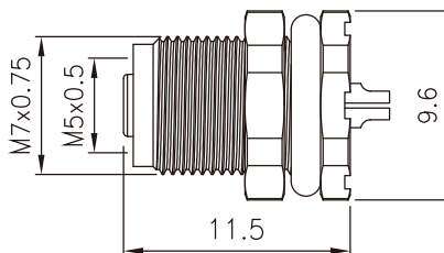
尺寸图 / Dimension
