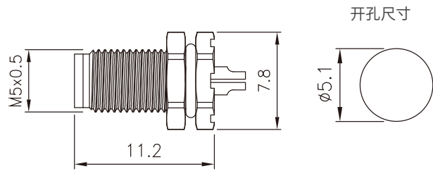
尺寸图 / Dimension
