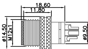
尺寸图 / Dimension
