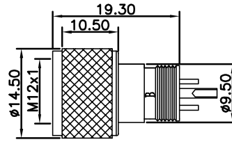
尺寸图 / Dimension
