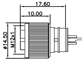
尺寸图 / Dimension
