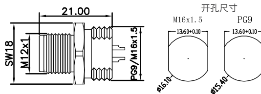
尺寸图 / Dimension
