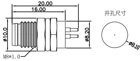
尺寸图 / Dimension
