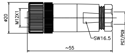
尺寸图 / Dimension
