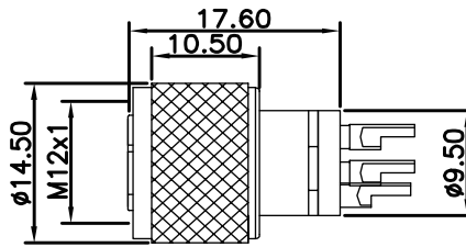
尺寸图 / Dimension
