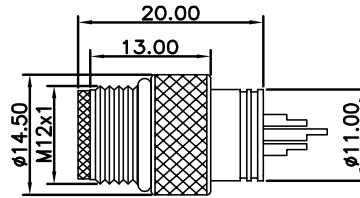
尺寸图 / Dimension
