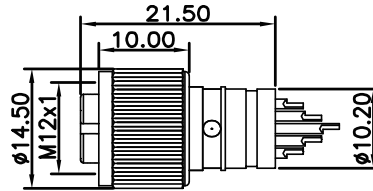
尺寸图 / Dimension
