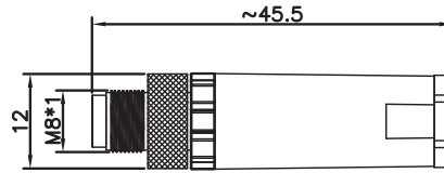
尺寸图 / Dimension
