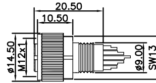
尺寸图 / Dimension
