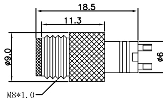
尺寸图 / Dimension
