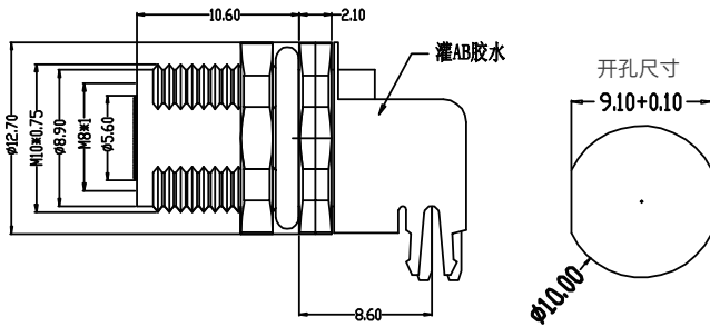
尺寸图 / Dimension
