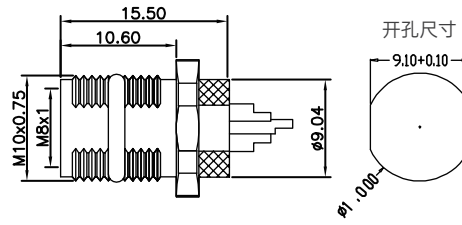
尺寸图 / Dimension
