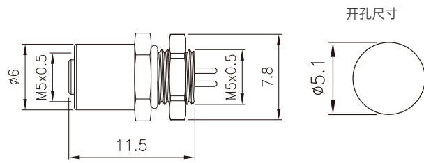
尺寸图 / Dimension
