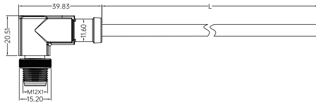
尺寸图 / Dimension
