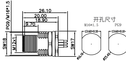
尺寸图 / Dimension
