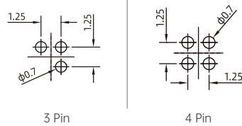
PCB芯位图 / PCB core diagram
