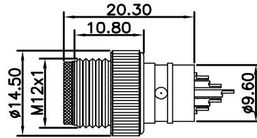
尺寸图 / Dimension
