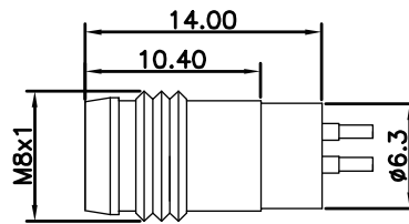
尺寸图 / Dimension
