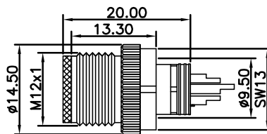
尺寸图 / Dimension
