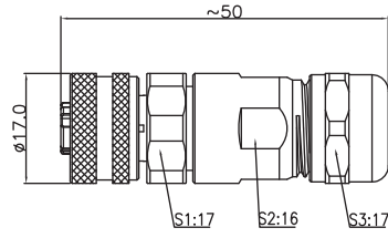
尺寸图 / Dimension
