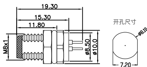
尺寸图 / Dimension
