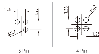
PCB芯位图 / PCB core diagram
