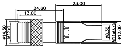
尺寸图 / Dimension
