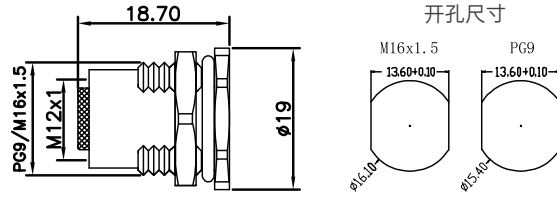
尺寸图 / Dimension
