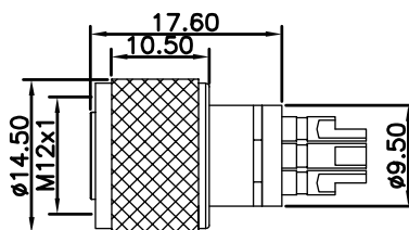
尺寸图 / Dimension
