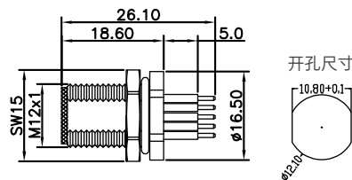
尺寸图 / Dimension
