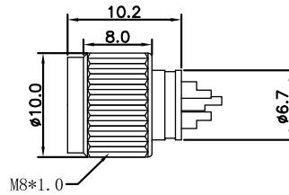
尺寸图 / Dimension
