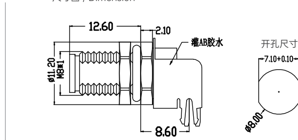
尺寸图 / Dimension
