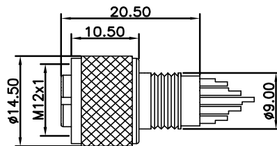
尺寸图 / Dimension
