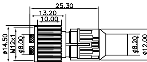
尺寸图 / Dimension
