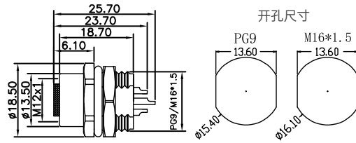
尺寸图 / Dimension
