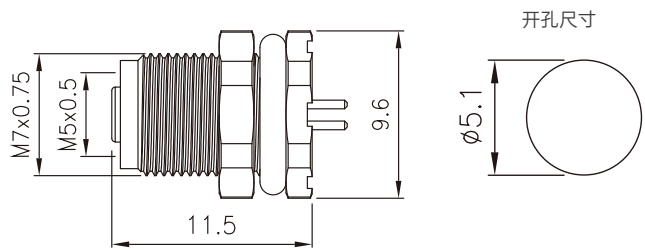
尺寸图 / Dimension
