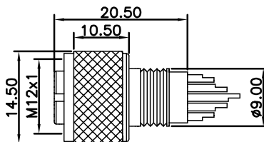
尺寸图 / Dimension
