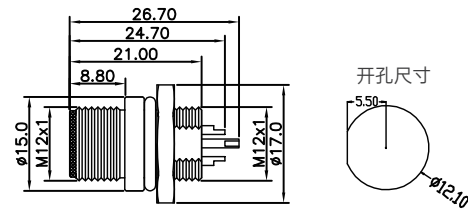
尺寸图 / Dimension
