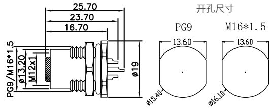
尺寸图 / Dimension
