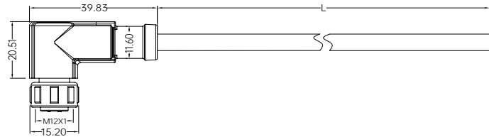
尺寸图 / Dimension
