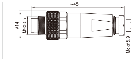
尺寸图 / Dimension
