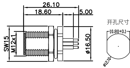
尺寸图 / Dimension
