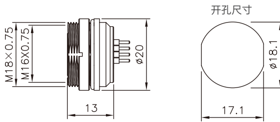
尺寸图 / Dimension
