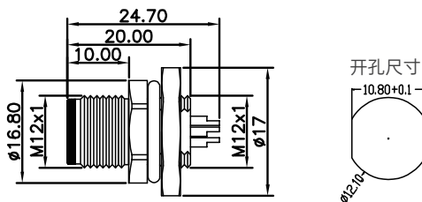
尺寸图 / Dimension
