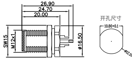
尺寸图 / Dimension
