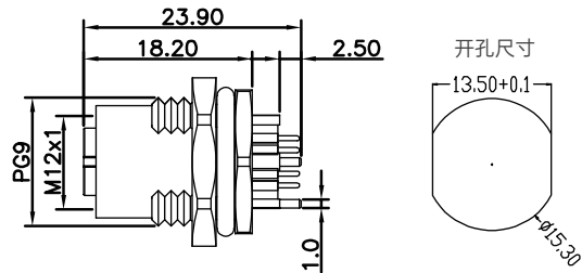
尺寸图 / Dimension
