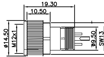
尺寸图 / Dimension
