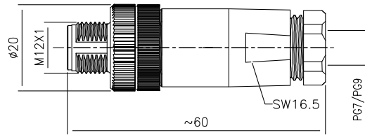
尺寸图 / Dimension
