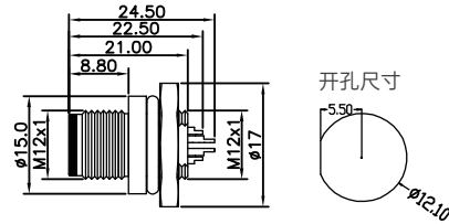
尺寸图 / Dimension
