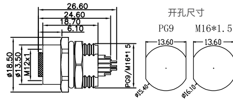
尺寸图 / Dimension
