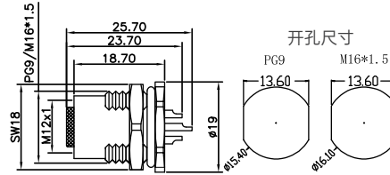
尺寸图 / Dimension
