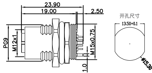
尺寸图 / Dimension
