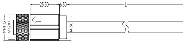
尺寸图 / Dimension
