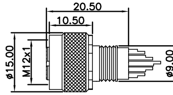
尺寸图 / Dimension
