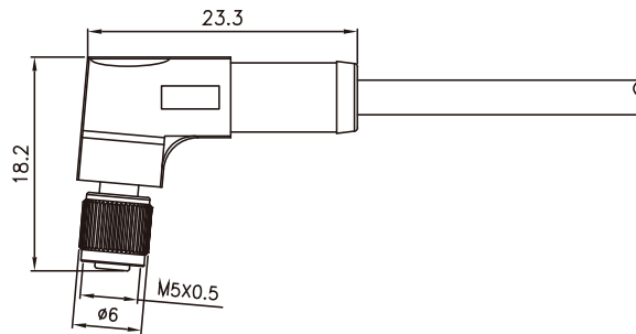
尺寸图 / Dimension
