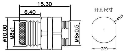
尺寸图 / Dimension
