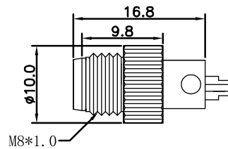
尺寸图 / Dimension
