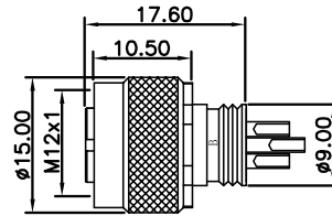
尺寸图 / Dimension
