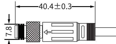
尺寸图 / Dimension
