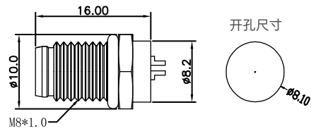
尺寸图 / Dimension
