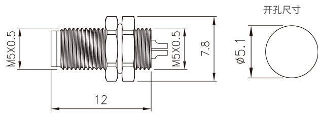
尺寸图 / Dimension
