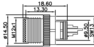
尺寸图 / Dimension
