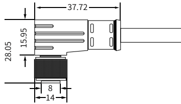
尺寸图 / Dimension
