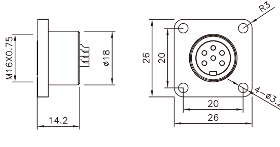
尺寸图 / Dimension
