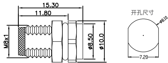
尺寸图 / Dimension
