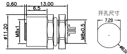
尺寸图 / Dimension
