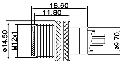
尺寸图 / Dimension
