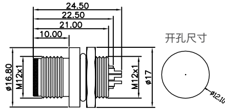
尺寸图 / Dimension
