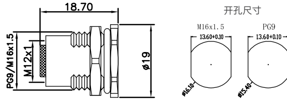
尺寸图 / Dimension
