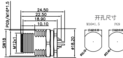
尺寸图 / Dimension
