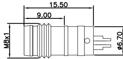
尺寸图 / Dimension
