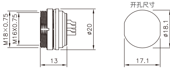
尺寸图 / Dimension
