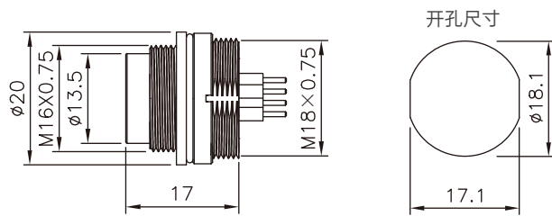
尺寸图 / Dimension
