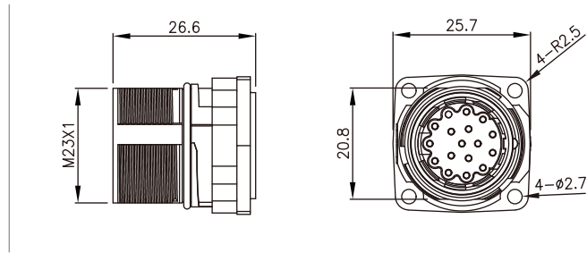
尺寸图 / Dimension
