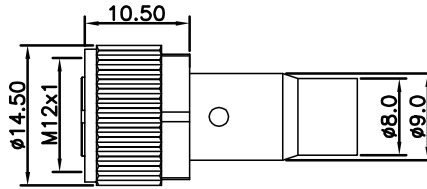
尺寸图 / Dimension
