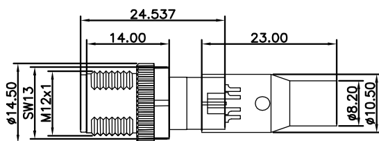
尺寸图 / Dimension
