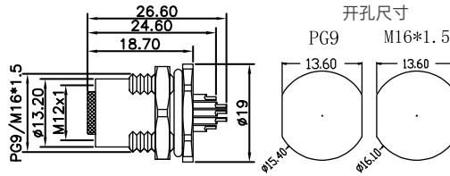
尺寸图 / Dimension
