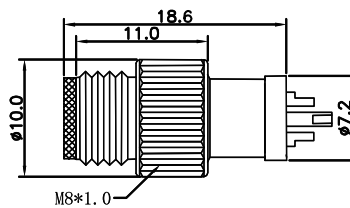
尺寸图 / Dimension
