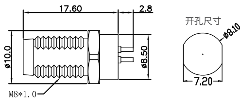
尺寸图 / Dimension
