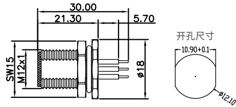
尺寸图 / Dimension
