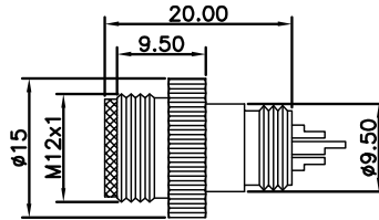
尺寸图 / Dimension
