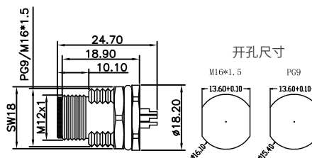
尺寸图 / Dimension
