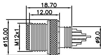
尺寸图 / Dimension
