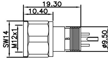
尺寸图 / Dimension
