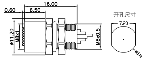
尺寸图 / Dimension
