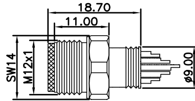
尺寸图 / Dimension
