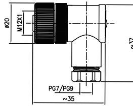
尺寸图 / Dimension
