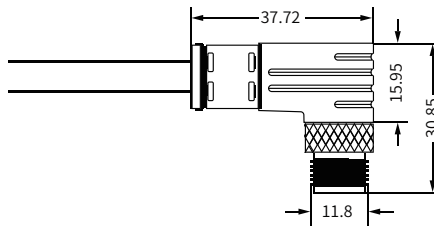
尺寸图 / Dimension
