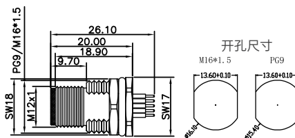
尺寸图 / Dimension
