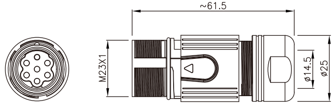
尺寸图 / Dimension
