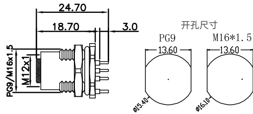
尺寸图 / Dimension
