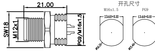
尺寸图 / Dimension
