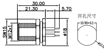
尺寸图 / Dimension
