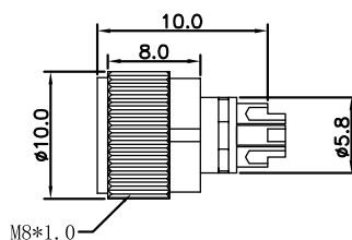
尺寸图 / Dimension
