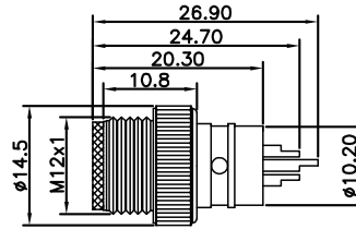
尺寸图 / Dimension
