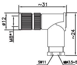
尺寸图 / Dimension
