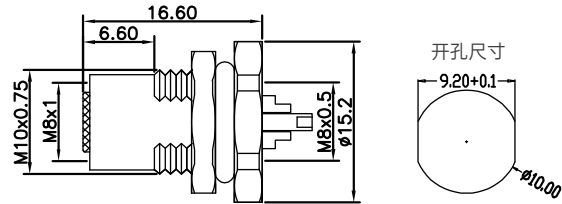
尺寸图 / Dimension
