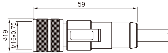
尺寸图 / Dimension
