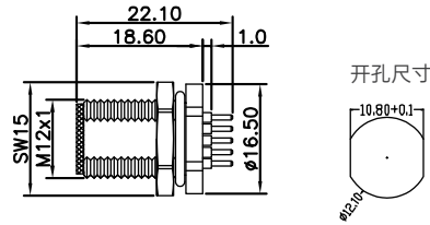
尺寸图 / Dimension
