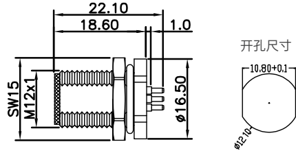
尺寸图 / Dimension
