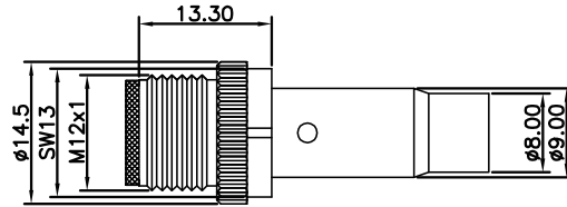
尺寸图 / Dimension
