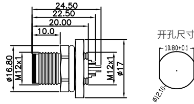
尺寸图 / Dimension
