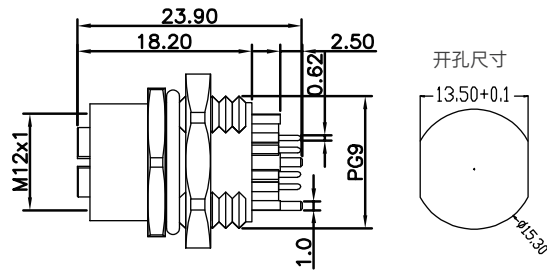
尺寸图 / Dimension
