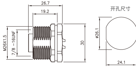
尺寸图 / Dimension
