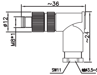
尺寸图 / Dimension
