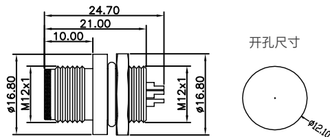
尺寸图 / Dimension
