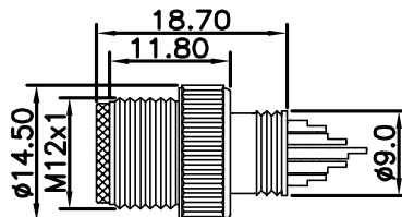
尺寸图 / Dimension
