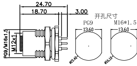
尺寸图 / Dimension
