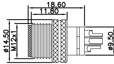
尺寸图 / Dimension
