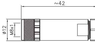
尺寸图 / Dimension
