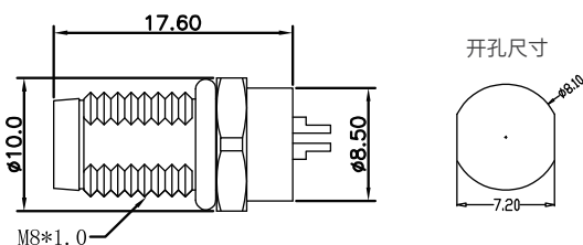
尺寸图 / Dimension
