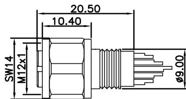
尺寸图 / Dimension
