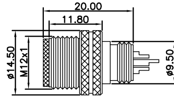
尺寸图 / Dimension
