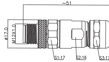
尺寸图 / Dimension
